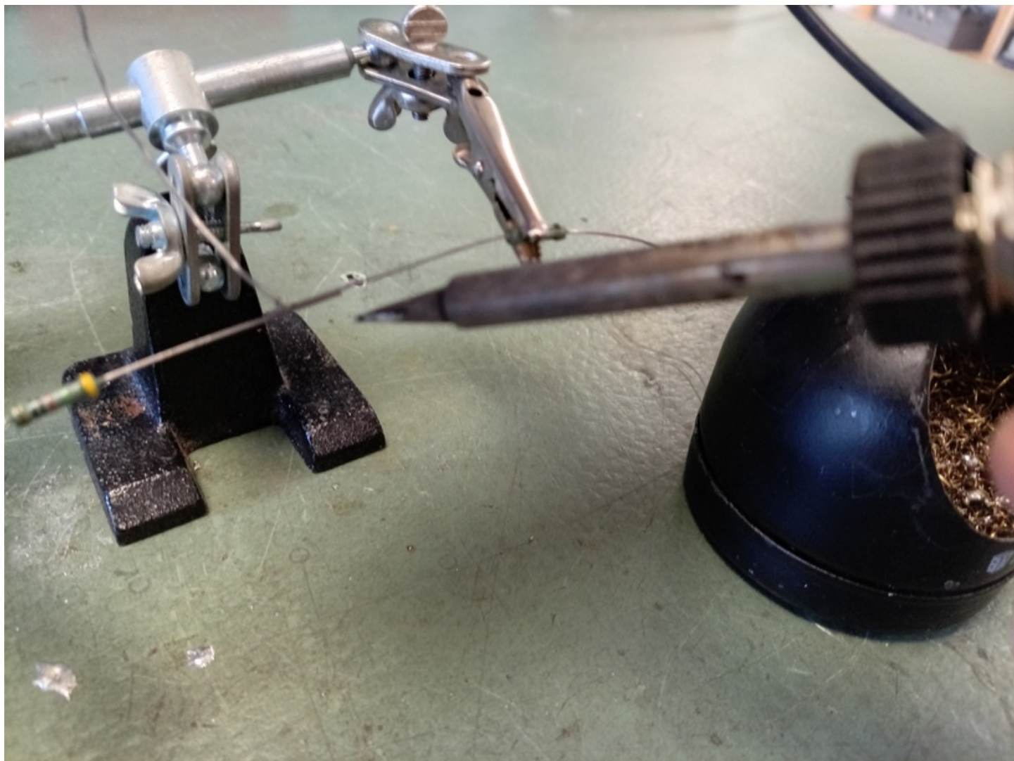
Figure 19: Sätt tänn till lödningsplatsen
