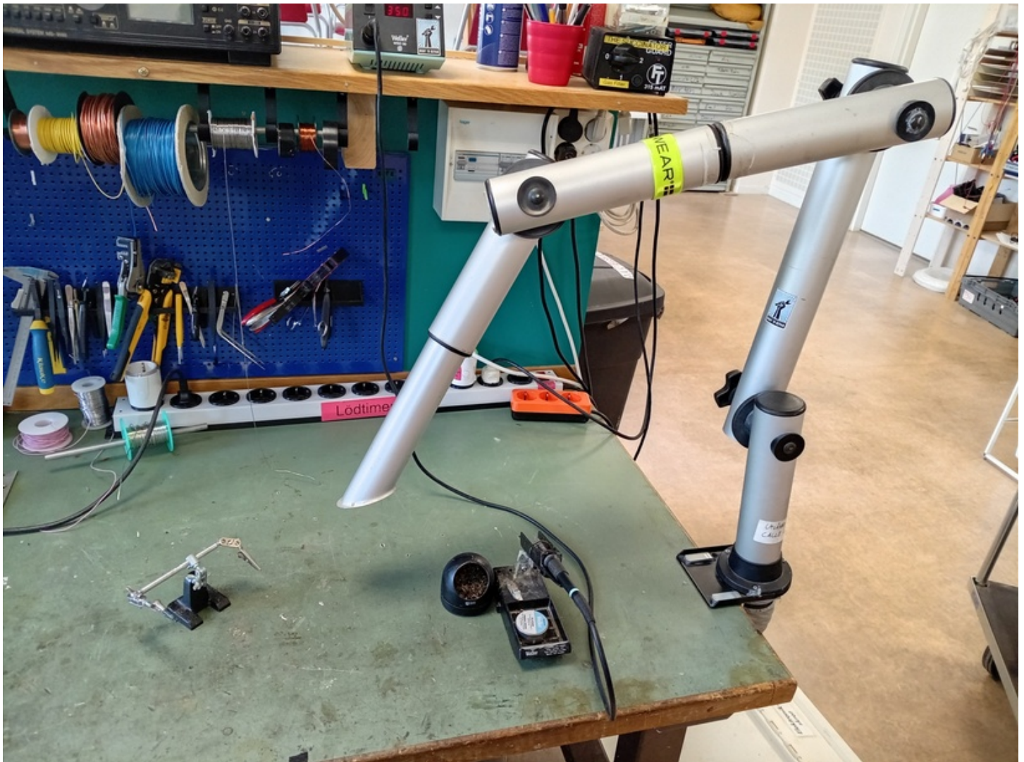
Figure 14: Sätt rökutsugsrör över bordet
